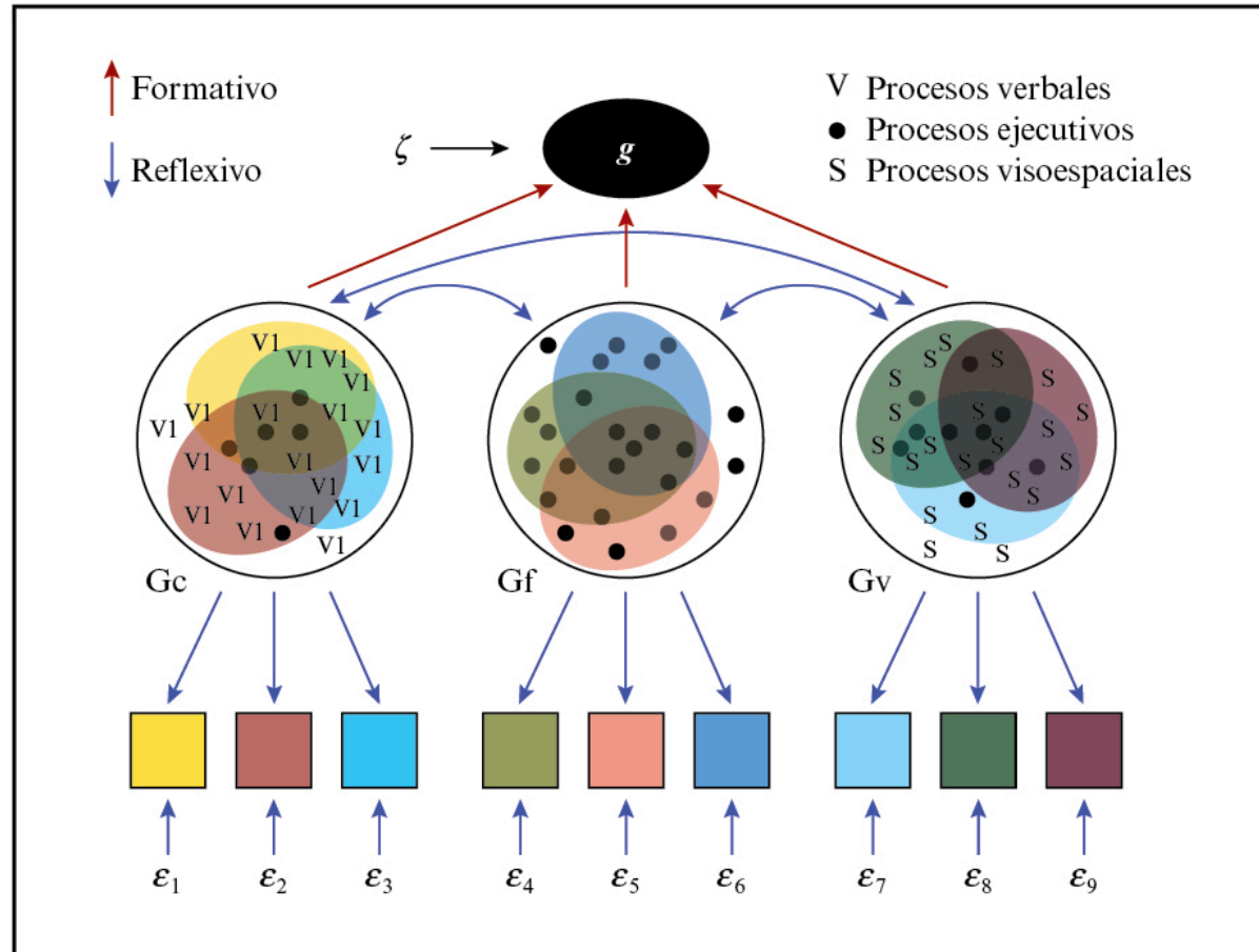
Figura 11.12**.—Una representación de la POT. Consiste en un modelo estructural híbrido, en parte formativo y en parte reflexivo. El segundo caso corresponde a un modelo oblicuo, pero también puede ajustar g como una variable latente formativa (la consecuencia común, en lugar de la causa común, de la correlación observada entre los factores de grupo). Se representa una versión sencilla centrándose solamente en G_c (inteligencia cristalizada), G_f (inteligencia fluida), G_v (inteligencia visoespacial) y procesos ejecutivos (Kovacs y Conway, 2016).
