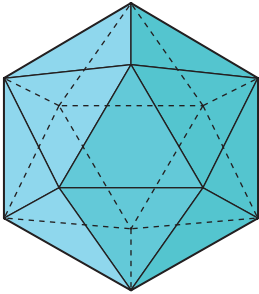
ICOSAEDRE
