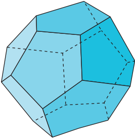
DODECAEDRE
