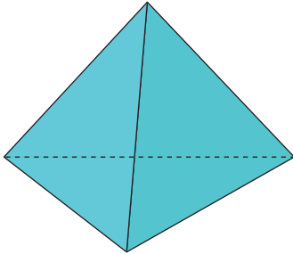
TETRAEDRE
