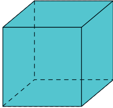
HEXAEDRE
