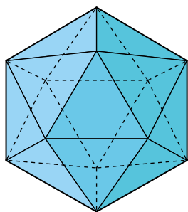
IKOSAEDROA
