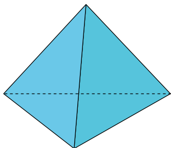
TETRAEDROA
