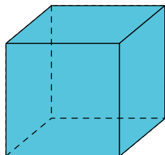
HEXAEDROA
