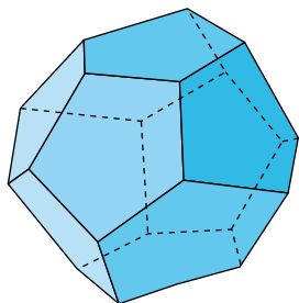
DODEKAEDROA
